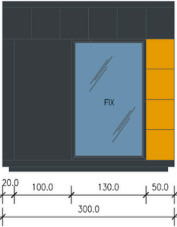
LEFT WALL
